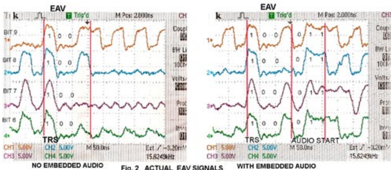
Fig. 2 ACTUAL EAV SIGNALS
